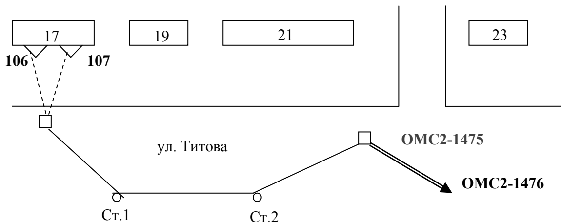
Рис. 6. Схема теодолитного хода
