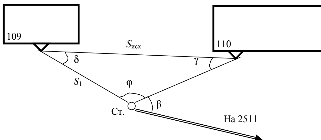
Рис. 9. Привязка съемочной станции к одинарным стенным знакам
