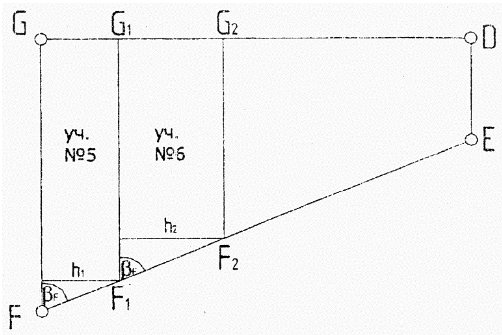
Рис. 2. Схема проектирования участков 5 и 6
