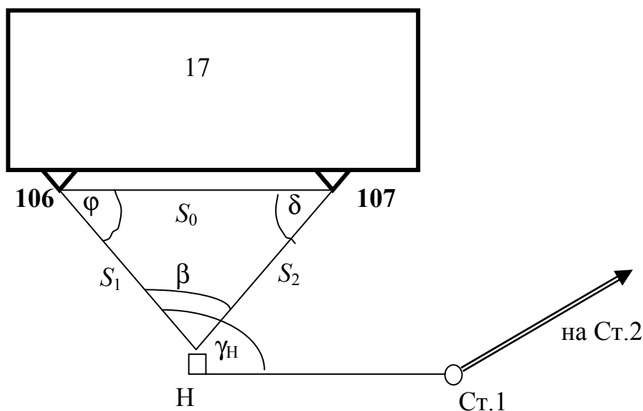
Рис. 8. Схема привязки хода к парным стенным знакам
