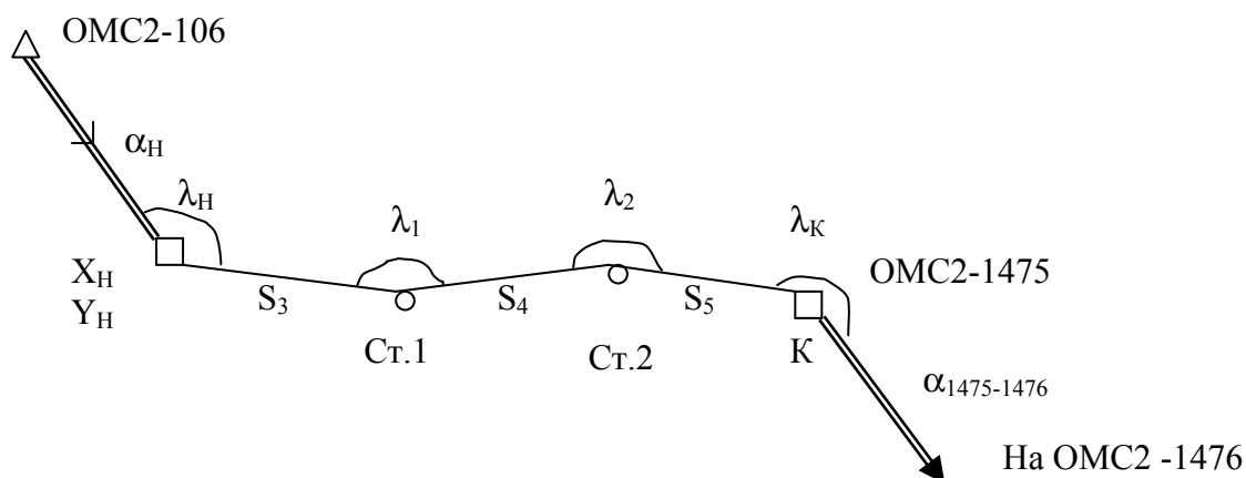
Рис. 9. Схема теодолитного хода
