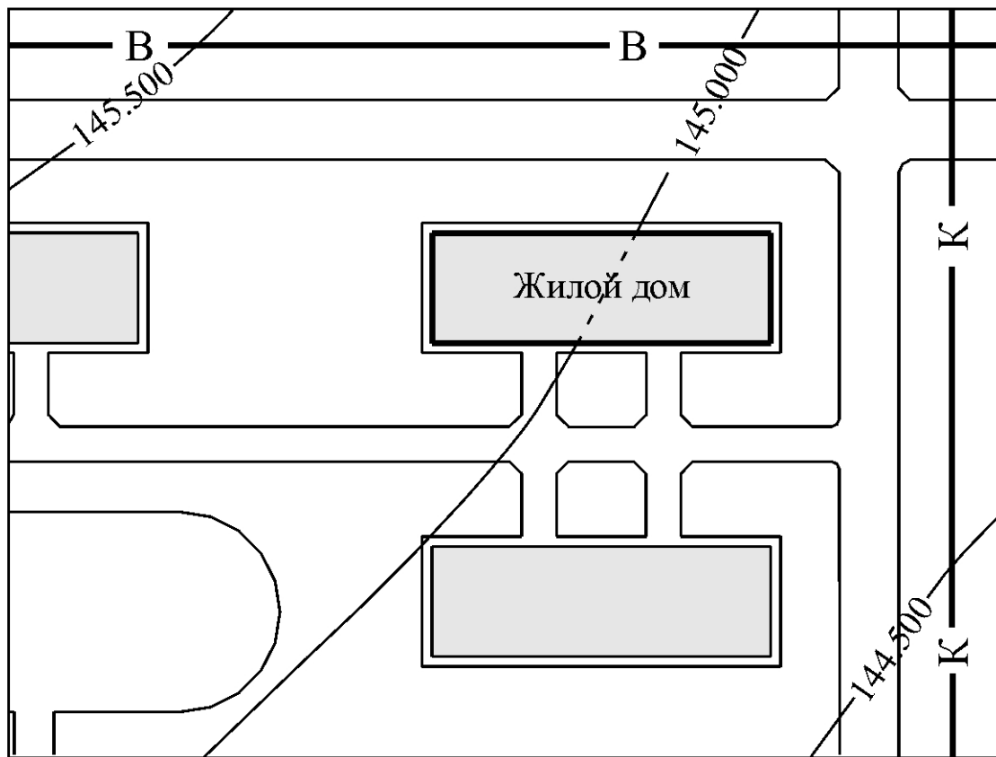
Вариант 14 – Генплан (1:1000)
