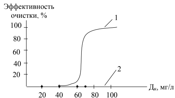
Рис. 7.3. Зависимость эффективности очистки сточной воды (раствор СЛ в 0,01 н NaOH) от дозы коагулянта (мг/л): 1 — Al_2(SO_4)_3 ; 2 — AlCl_3 .
