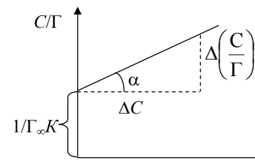
Рис.8.2. Уравнение Ленгмюра в линейной форме
