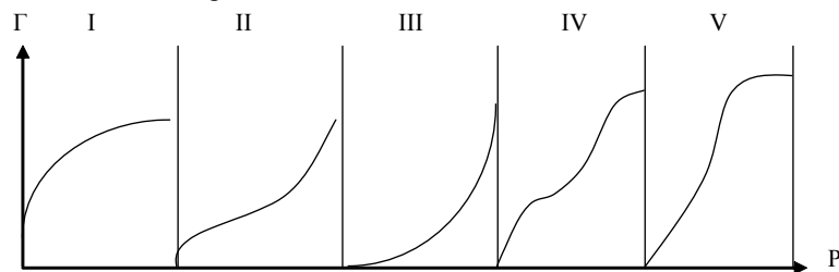
Рис. 8.3. Пять основных типов экспериментальных изотерм адсорбции газов и паров
