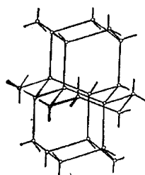
Рис. 1.3. Схема объемной структуры льда
