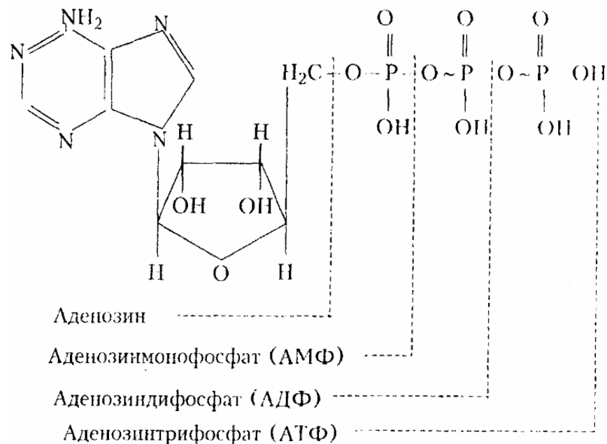
Рис. 13.2. Структура аденозинтрифосфата (АТФ).
