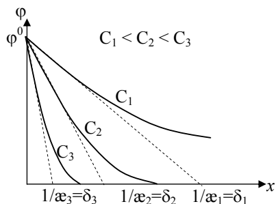
Рис. 7.2. Строение ДЭС
