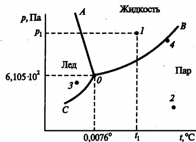
Рис.1.4. Диаграмма состояния воды в области невысоких давлений
