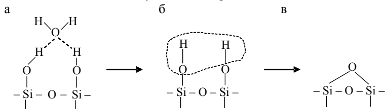
Рис. 8.4. Адсорбция воды на кремнеземе:
