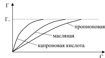
Рис. 8.1. Изотермы адсорбции
