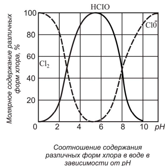
Рис. 6.1. Соотношение содержания различных форм хлора в воде в зависимости от pH
