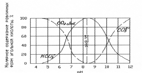
Рис.3.1. Зависимость содержания различных форм угольной кислоты от pH
