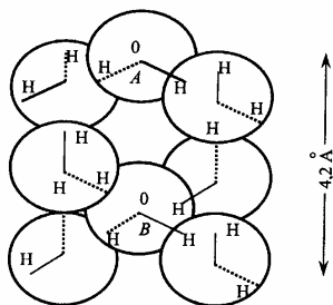
Рис. 1.1. «Кварцевая» структура воды
