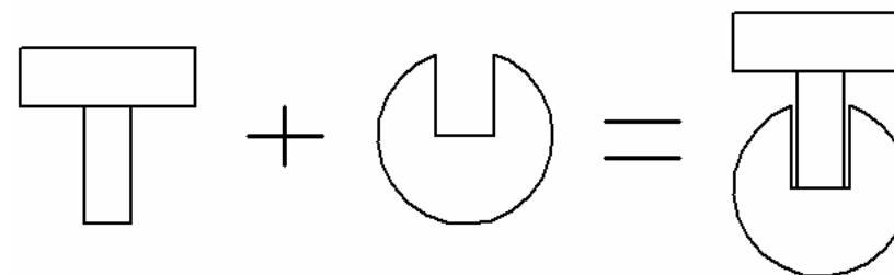
Рис.13.1. Образование комплекса между ферментом и субстратом
