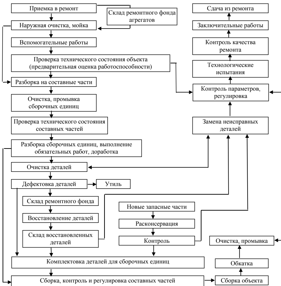
Рис. 1. Схема технологического процесса выполнения ремонта автомобилей [5]
