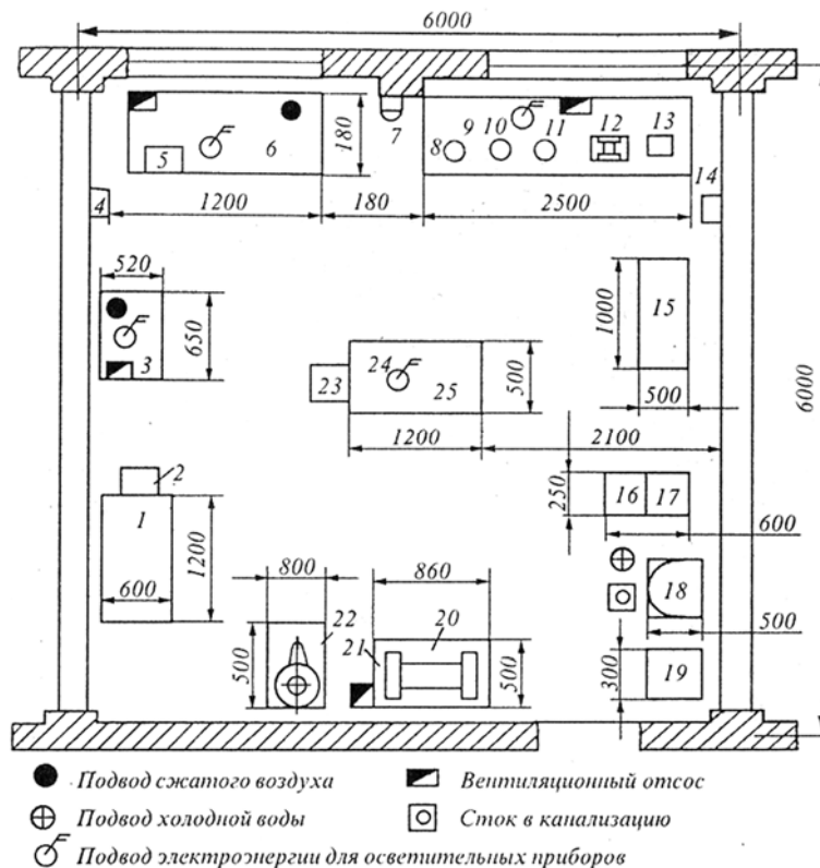
Рис. 1. Планировка рабочего места:
