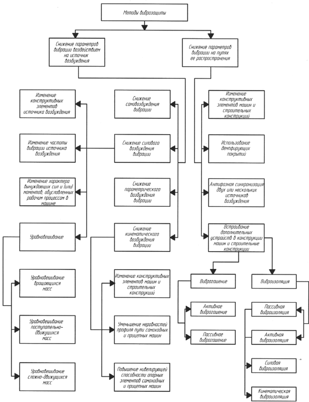
Рис. 6.1. Рекомендуемые методы снижения вибрации
