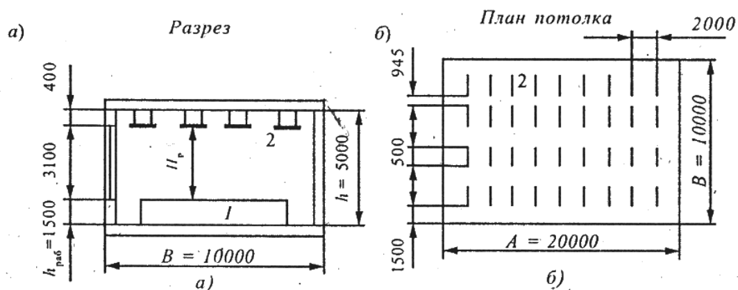
Рис. 10.2. Эскиз разреза и плана потолка с примерной схемой размещения люминесцентных ламп: 1 – столы; 2 – светильники
