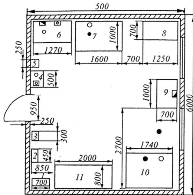
Рис 4. Планировка рабочего места медника:
