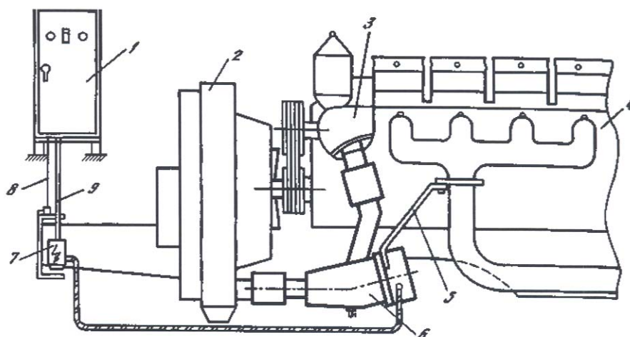
Рис. 2. Схема электроподогрева двигателей автомобилей:
