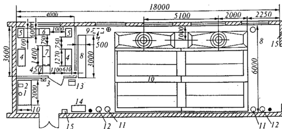
Рис. 6. Планировка рабочего места маляра:
