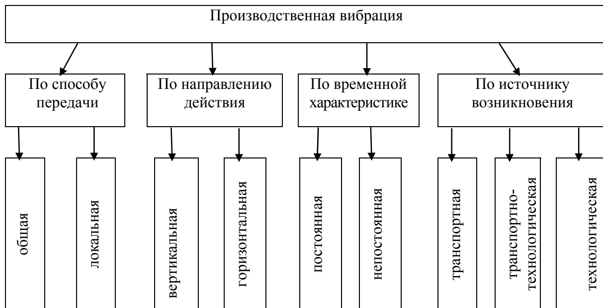
Рис. 5.1. Классификация производственной вибрации
