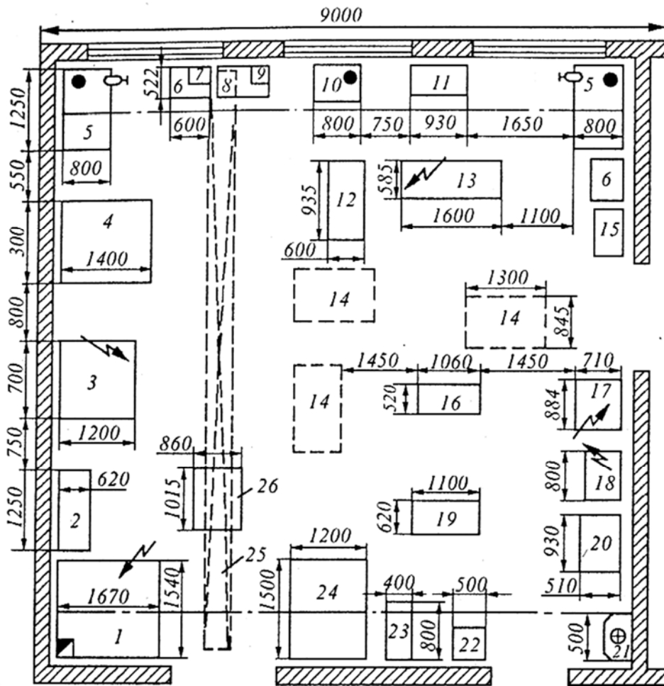
Рис. 8. Планировка рабочего места слесаря по ремонту двигателей: 1 – моечная установка для мойки блоков цилиндров; 2 – моечная ванна для деталей; 3 – станок для расточки цилиндров двигателей; 4 – станок для полирования цилиндров двигателей; 5 – слесарный верстак с пневматикой; 6 – инструментальная тумбочка; 7 – прибор для проверки и правки шатунов; 8 – шкаф для деталей шатунно-поршневой группы; 9 – прибор для определения упругости пружин клапанов и поршневых колец; 10 – стэнд для прессовки поршневых пальцев; 11 – стеллаж для приборов и приспособлений; 12 – станок для шлифования клапанов; 13 – станок для притирки клапанов; 14 – стэнд для ремонта двигателей; 15 – шкаф для деталей газораспределительного механизма; 16 – стэнд для сборки и разборки головок цилиндров двигателей; 17 – стэнд для обкатки и испытания компрессоров; 18 – стэнд для испытания масляных насосов и масляных фильтров; 19 – конторский стол; 20 – стеллаж для масляных и водяных насосов и компрессоров; 21 – умывальник; 22 – ящик для отходов; 23 – ларь для обтирочных материалов; 24 – стеллаж для двигателей; 25 – кран-балка; 26 – стэнд для разборки двигателей
