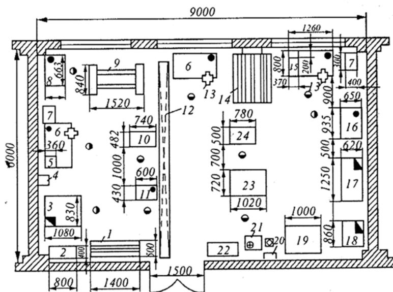
Рис. 7. Планировка рабочего места слесаря по ремонту агрегатов:
