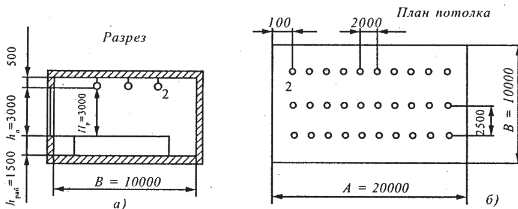
Рис. 10.1. Эскиз разреза и плана потолка с примерной схемой размещения светильников типа Люцетта: 1 – столы; 2 – светильники
