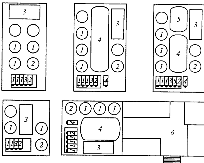
Рис. 7.1. Варианты компоновки передвижных мастерских для ТО и ремонта СДМ:
