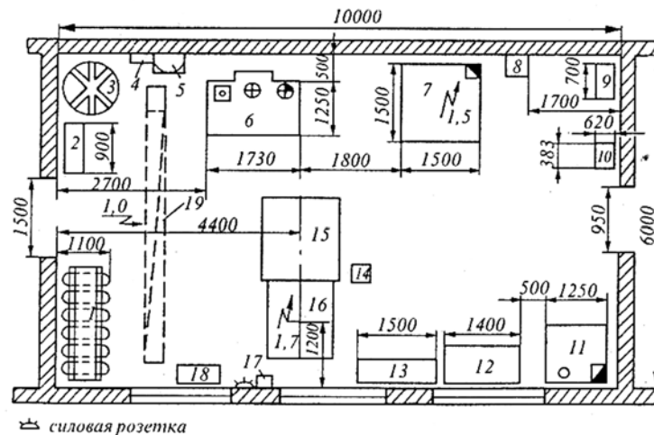
Рис 5. Планировка рабочего места шиномонтажника:
